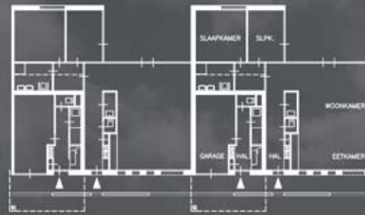
BEGANE GROND
